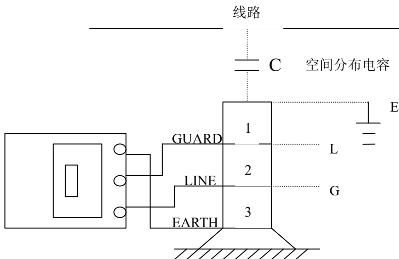
图 5 利用屏蔽端屏蔽干扰
