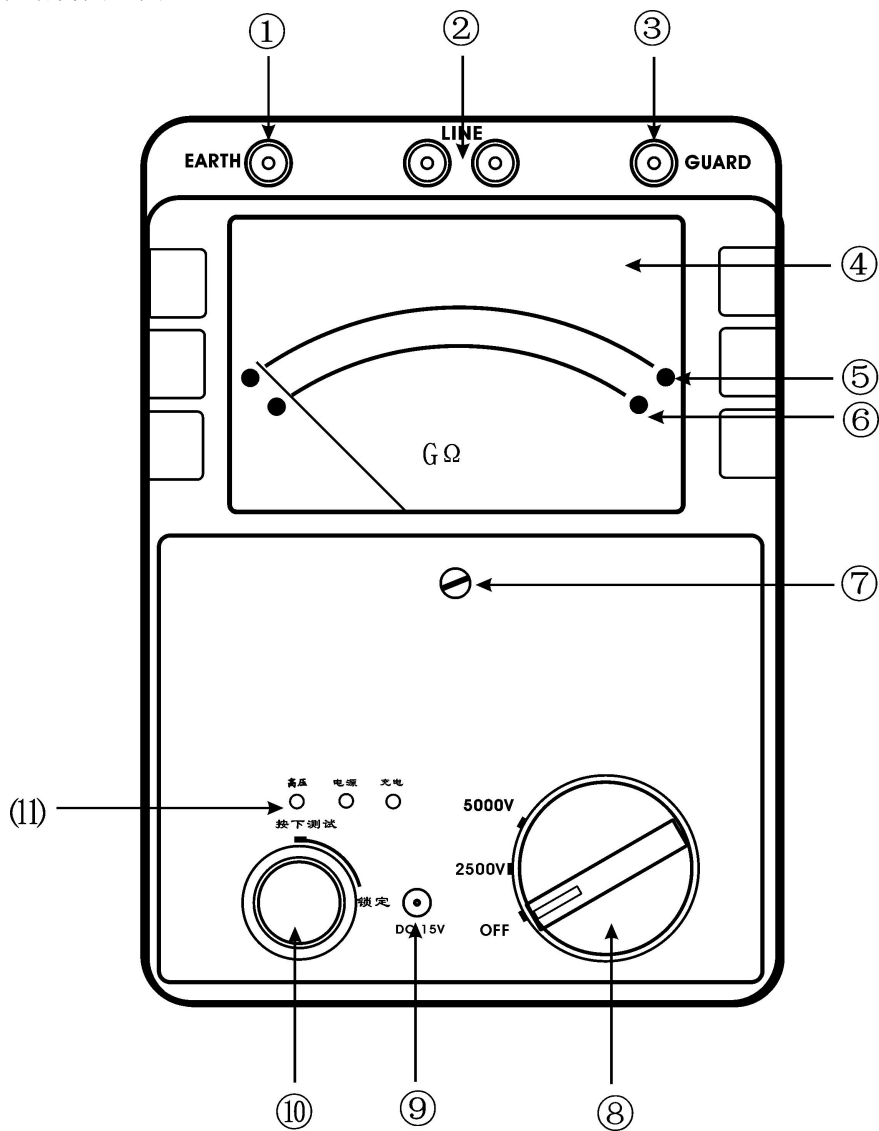
图 1：绝缘表结构图
