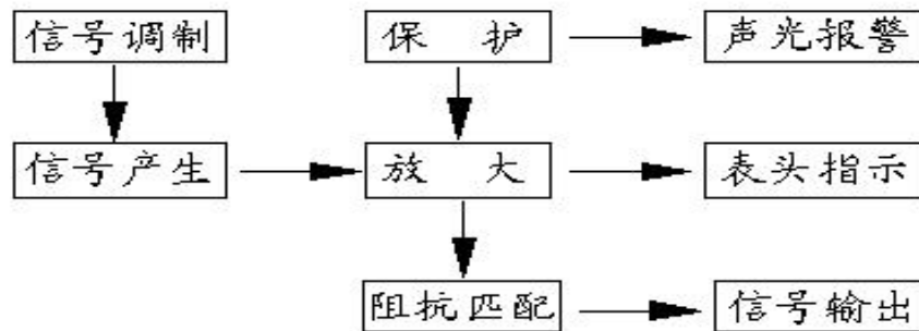
图 5. 路径仪方框图
