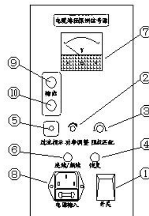
图 6. 路径仪面板图
