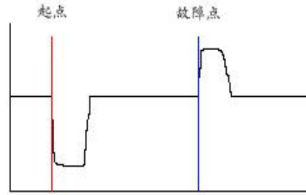
低阻〔短路〕故障波形及定位
