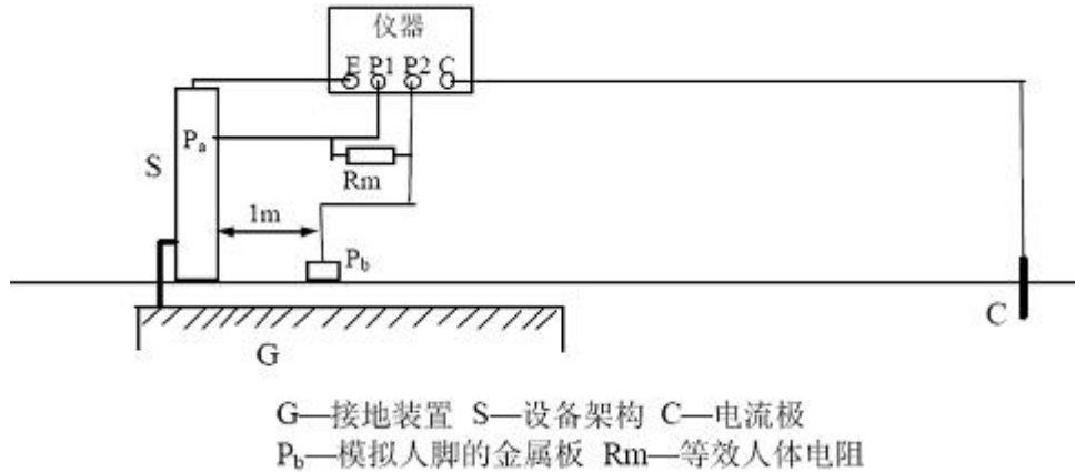
图5 接触电压测量接线图
