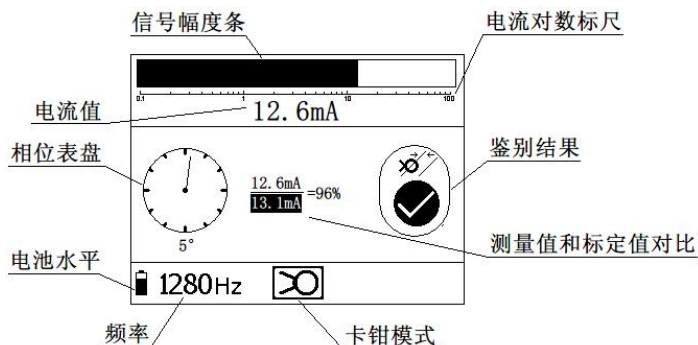
图 5-1-2 卡钳鉴别界面
