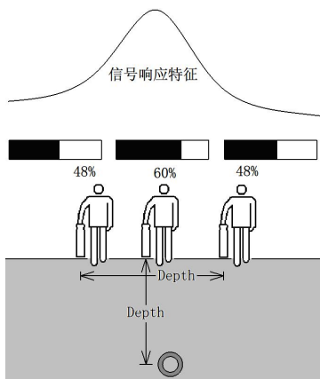
图 4-4-4 宽峰 80%法测深
