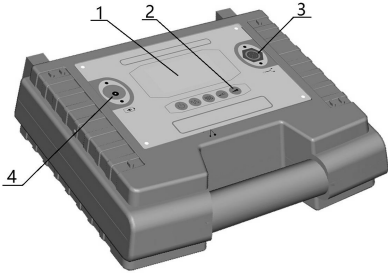
图 1-4-1 发射机整体
