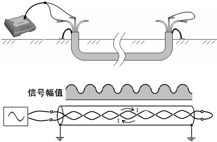
图 3-1-5 相间接法
