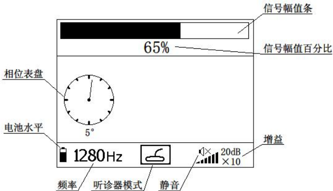
图 5-1-2 听诊器界面
