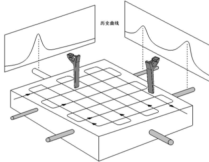
图 4-2-1 无源法区域探查
