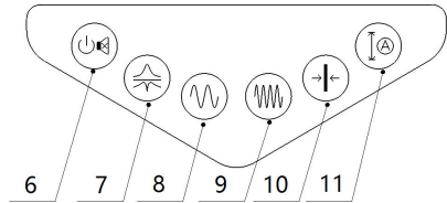
图 1-5-2 接收机键盘
