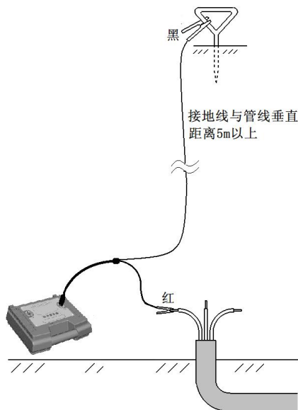
图 6-1-1 接地故障定点接线
