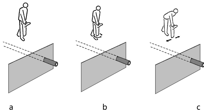
图 4-3-1 精确定位
