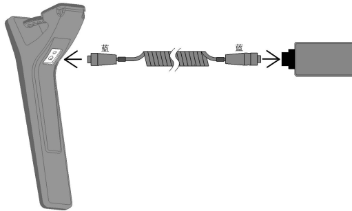
图 5-1-4 听诊器连接
