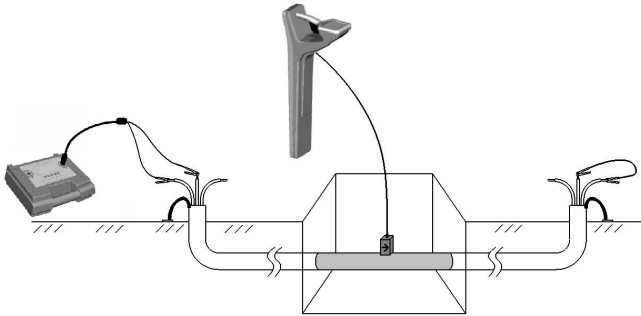
图 5-1-3 听诊器鉴别
