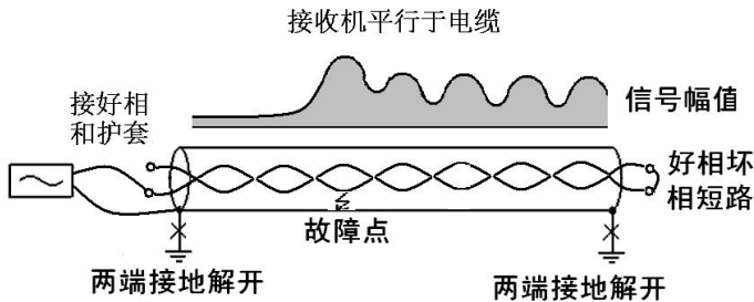
图7-2-1 相对铠装接地故障定点
