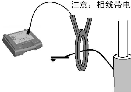
图 3-2-2 运行电缆卡钳耦合法 2 (卡电缆接地线)
