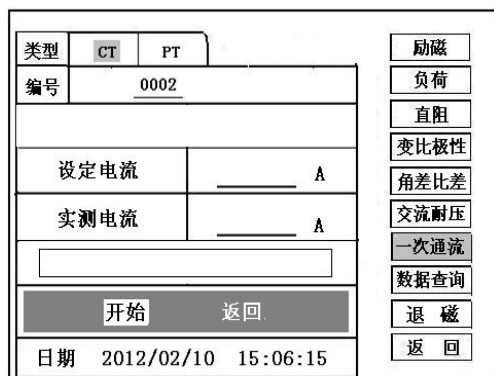
图 16、CT 一次流测试界面
