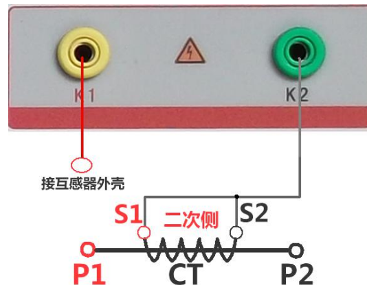
图 19, CT 交流耐压接线图
