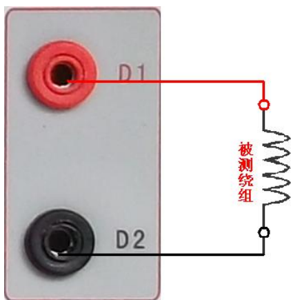
图 24, 直阻测试接线图
