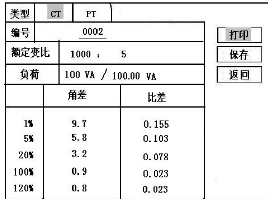
图 15, CT 角差比差测试结果界面
