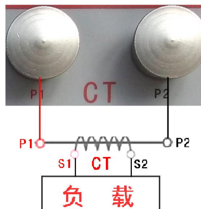
图 17、CT 一次通流接线图
