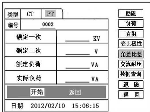
图 30，PT 角差比差测试界面
