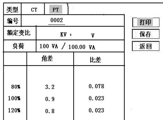
图 31，PT 角差比差测试结果界面
