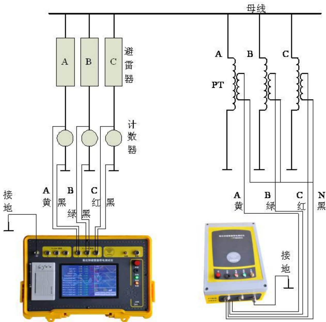
图 3 测试线接线示意图
