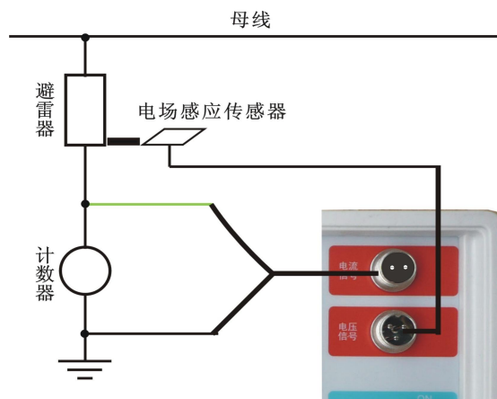
图 4 感应模式测试接线示意图
