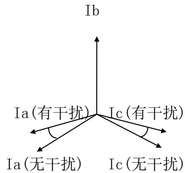
图 12 AC 相受 B 相影响
