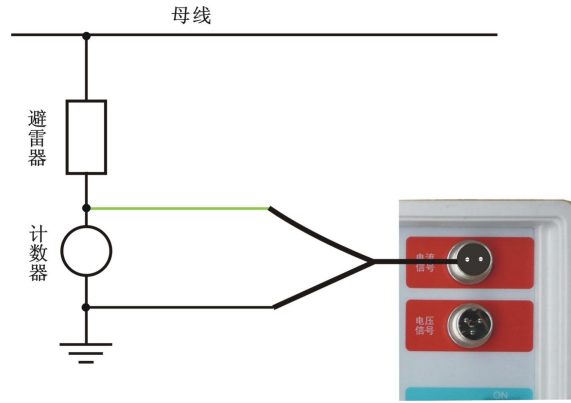
图 3 无线模式(测试相序: B)测量接线示意图
