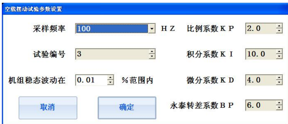
图 4.1 空载摆动试验参数设置
