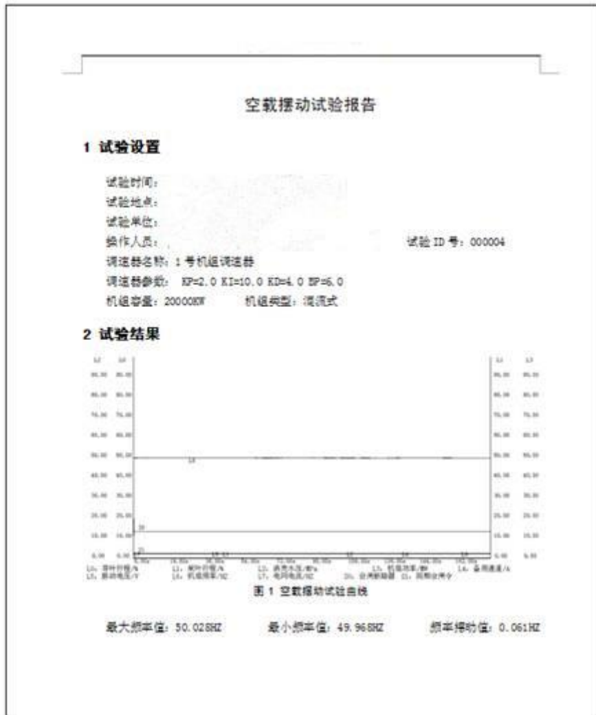
图 3.9 空载摆动试验报告
