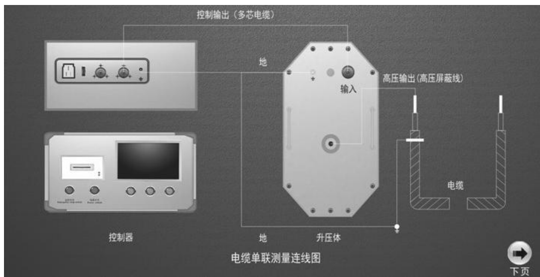
图 4a VLF-30/1.1 (连线图)
