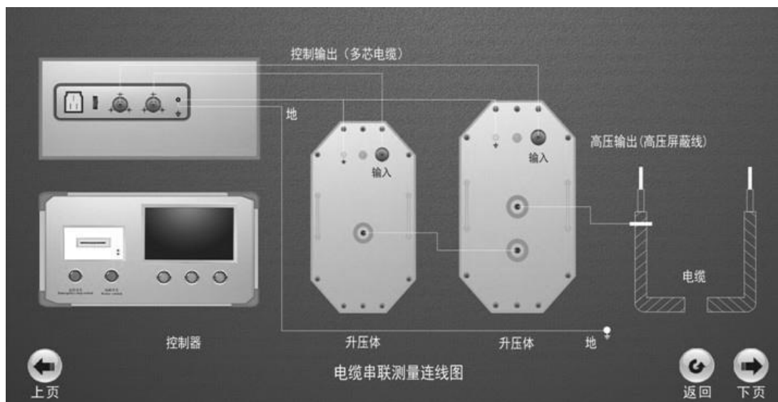
图 4b VLF-80/1.1 (连线图)
