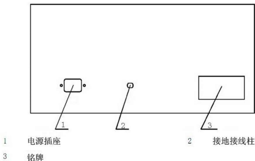
图 3 后板
