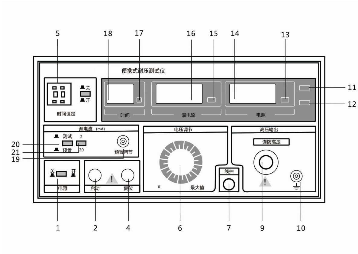
图 2 面板
