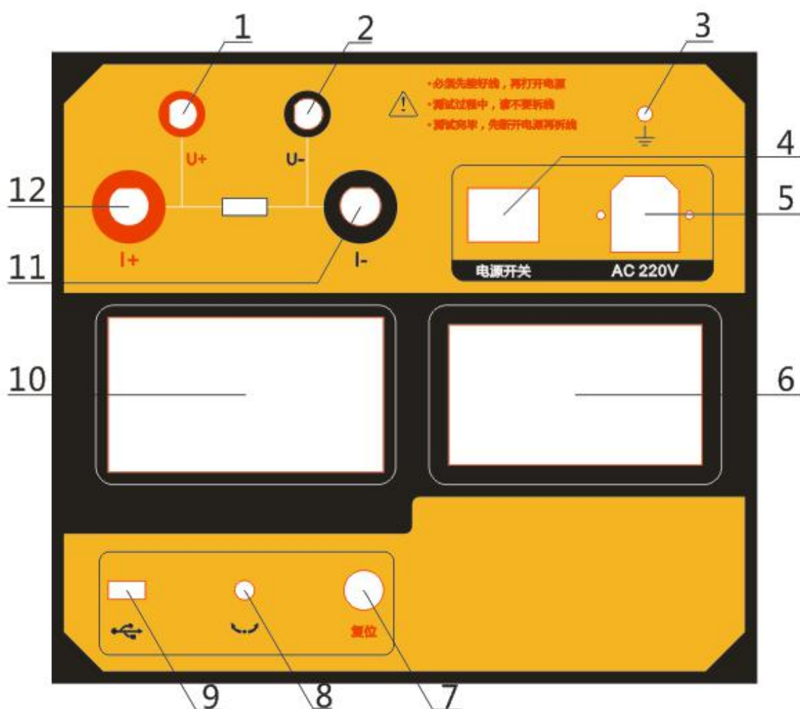
图 1 面板布局图
