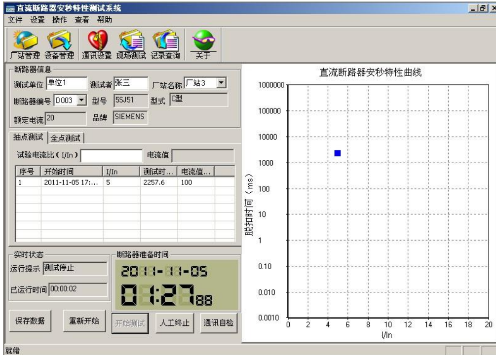
图 23 抽点测试
